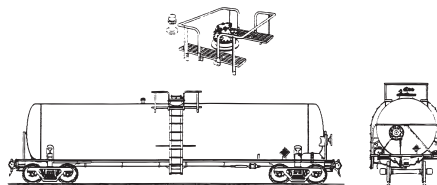
Carrotanque de baja presión para líquidos
